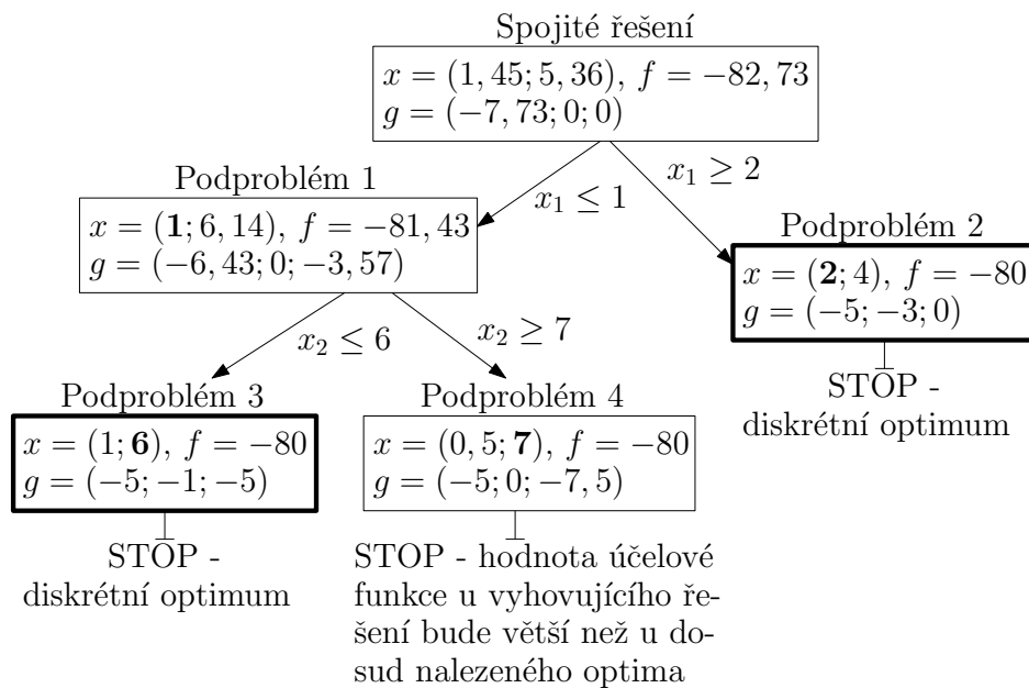
Obrázek 4.4: Metoda větví a mezí s kombinací spojitých a diskretních proměnných
