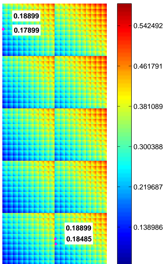
Obrázek D.1: Hypergraf pětiprutové konstrukce s vykreslením všech hmotností pro celou úlohu a zakreslením 4 nejlepších řešení (legenda v lb), liché proměnné jsou svisle, sudé jsou vodorovně, 1. proměnná tvoří dva sloupce
