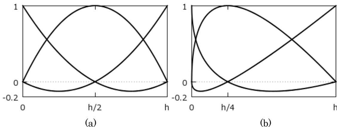
Obrázek 4.16: Bázové funkce (a) pro klasické, (b) pro upravené kvadratické prvky
