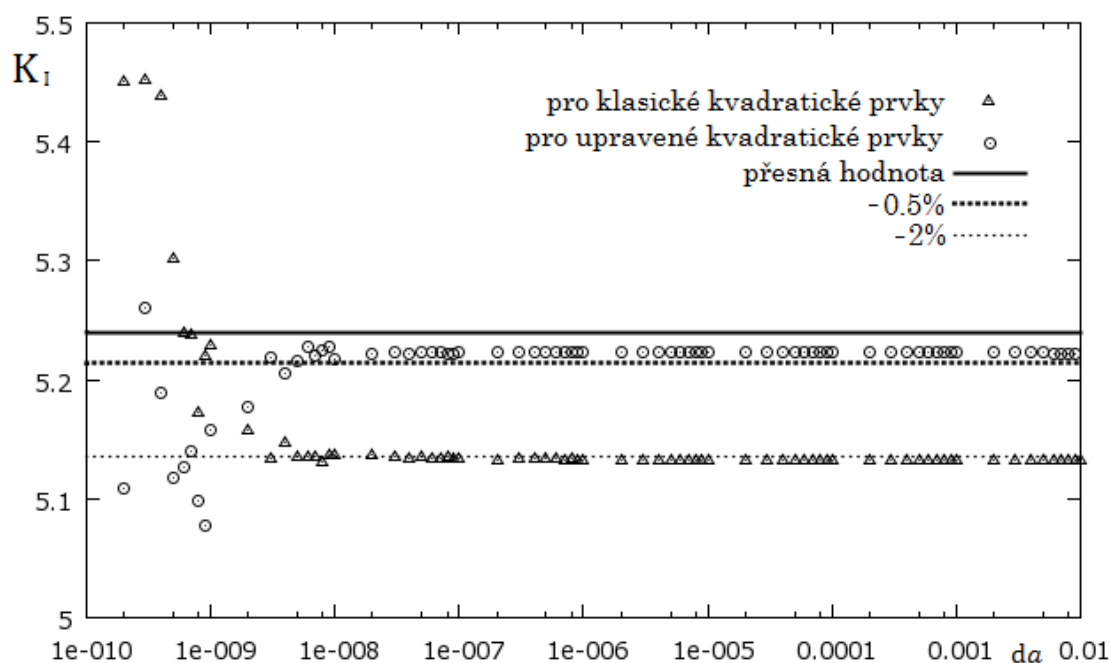
Obrázek 4.20: K_I vypočtený pomocí globální energetické metody pro různě velké zvětšení trhliny da , s použitím kvadratických prvků, porovnání klasických a upravených kvadratických prvků
