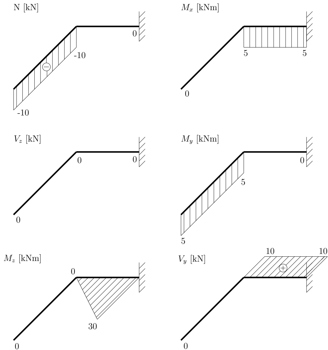
Obrázek 3: Vykreslení vnitřních sil
