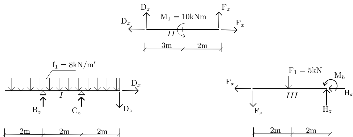
Obrázek 2: Rozdělení konstrukce na jednotlivé desky.
