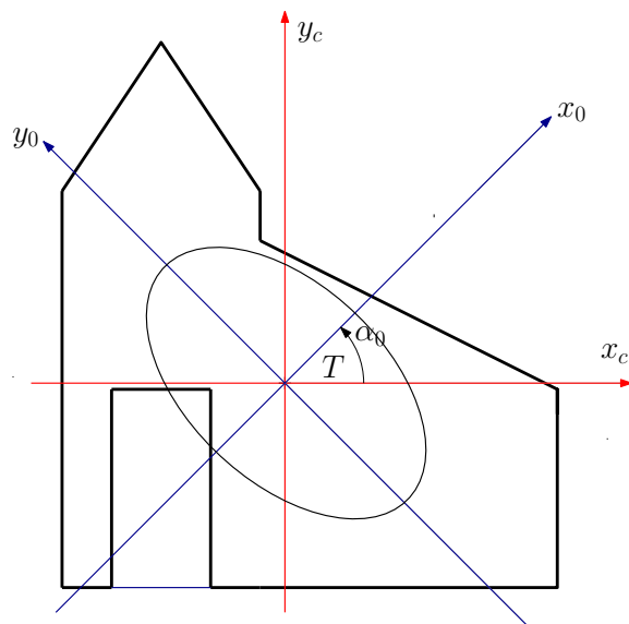
Obrázek 4: Elipsa setrvačnosti.
